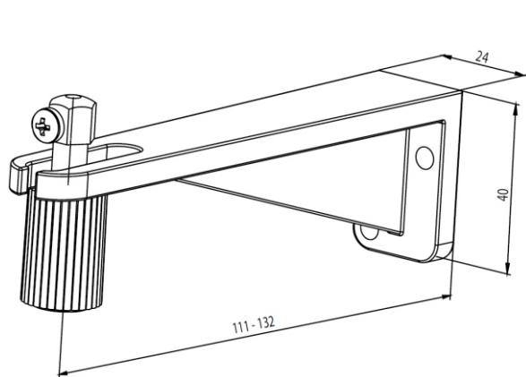
Držák č.5
