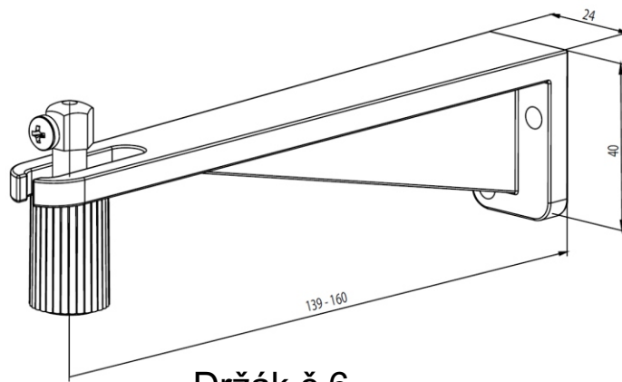
Držák č.6
